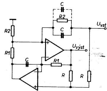
Obr. 4. Pásmová zádrž (ekvalizér) druhého stupně
